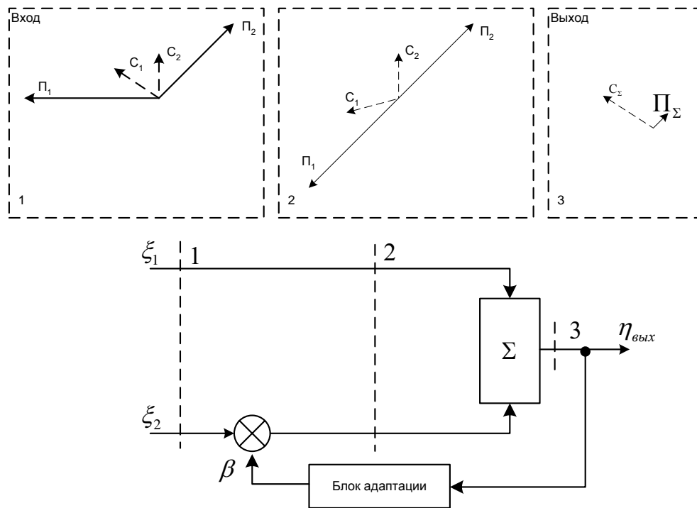
Рис. 1. Пространственная обработка сигнала
