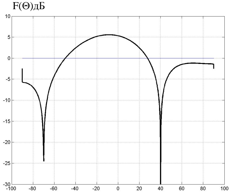
Рис.3. Сечение диаграммы направленности плоскостью Y = 0 ,
